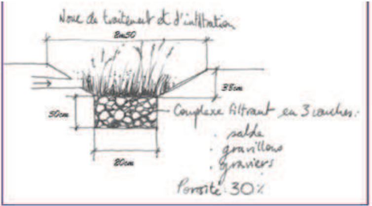
Figure 11 : Coupe d'une noue (source : dossier loi sur l'eau, p.73)
